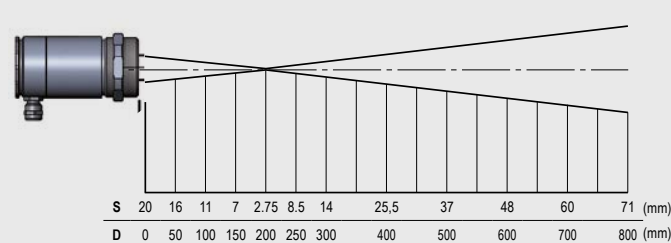
CF3 optics 75:1
