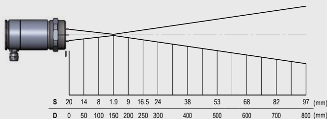
CF2 optics 75:1
